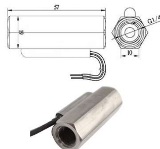
Delicate SUS Circulation Air Flow Switch
